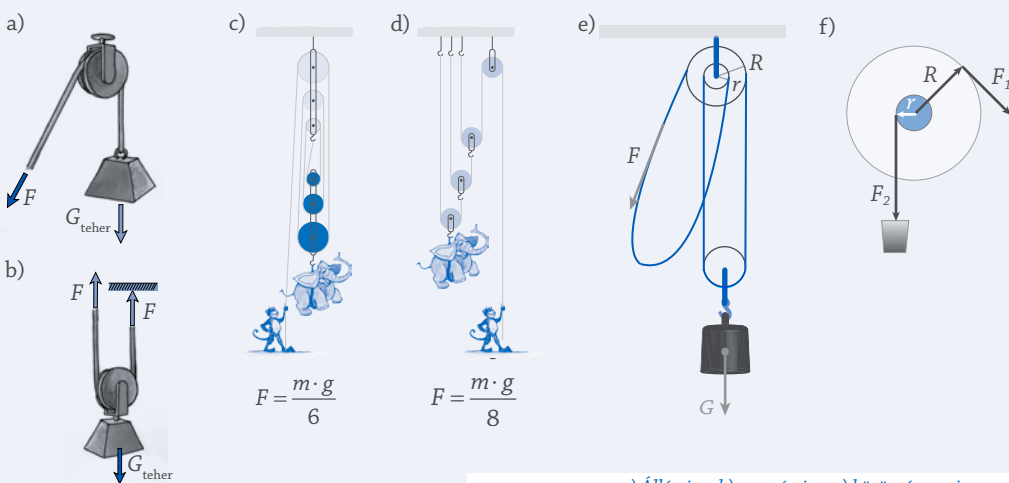
a) Állócsiga, b) mozgócsiga, c) közönséges csigasor, d) Arkhimédészi csigasor, e) differenciális csigasor, f) a hengerkerék
