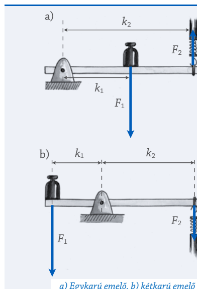
a) Egykarú emelő, b) kétkarú emelő
