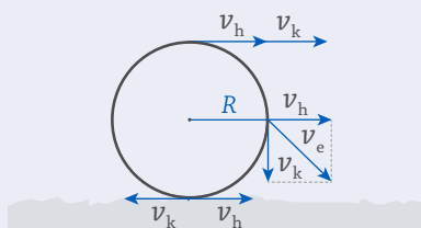
Tisztán gördülő test kerületi pontjainak sebessége
