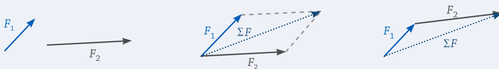
Szöveget bezáró erők összegzése paralelogramma- és háromszögmódszerrel
