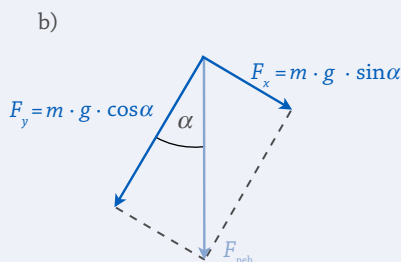
a) A dobozra három erő hat b) Bontsuk fel a nehézségi erőt!
