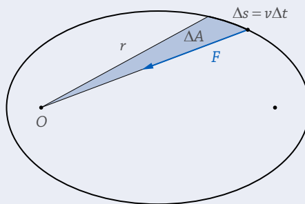
Bolygó mozgása a Nap körül
