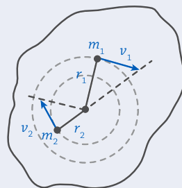
Tehetlenségi nyomaték meghatározása
