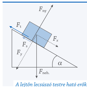
A lejtőn lecsúszó testre ható erők
