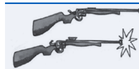
„Visszarúg” a fegyver
