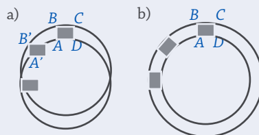
a) Haladó mozgás körpályán, b) haladó és forgó mozgás összetétele
