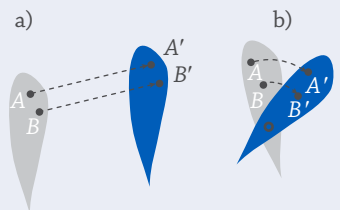
a) A haladó és b) forgó mozgást végző test pontjainak pályája
