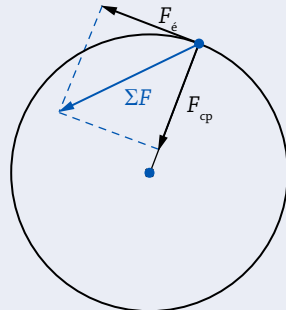
Változó forgómozgást végző test pályájának egy adott pontjában ható erők
