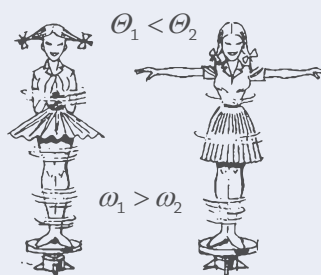
A perdületmegmaradás szemléltetése
