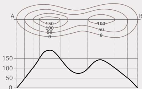
A metszetszerkesztés lépései
